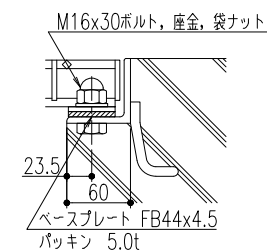
ボルト固定 詳細図
