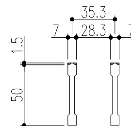
ベアリングバー 詳細図
