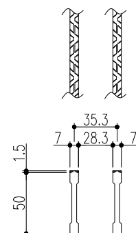
ベアリングバー 詳細図
