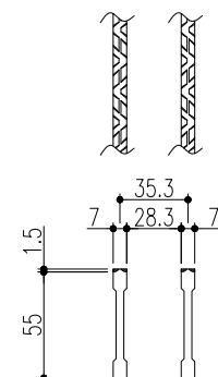
ベアリングバー 詳細図
