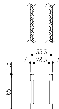
ベアリングバー 詳細図
