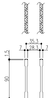
ベアリングバー 詳細図
