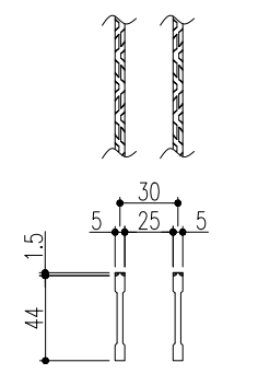
ベアリングバー 詳細図
