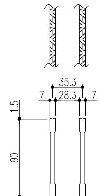
ベアリングバー 詳細図
