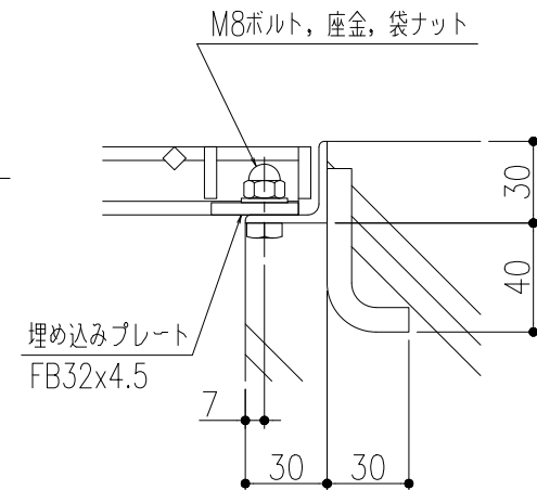
ボルト固定 詳細図
