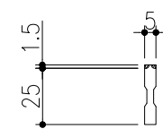
ベアリングバー 詳細図
