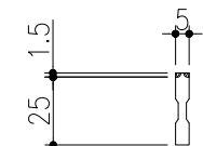
ベアリングバー 詳細図
