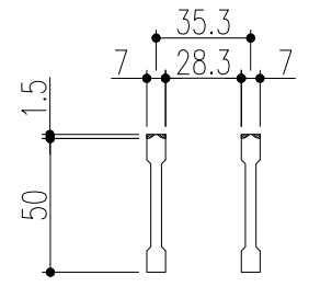
べアリングバー 詳細図
