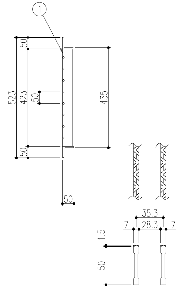
ベアリングバー 詳細図
