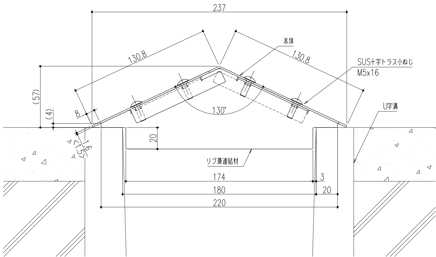
断面詳細図 S=1/2 ※＜＞寸法はSYGCです。
