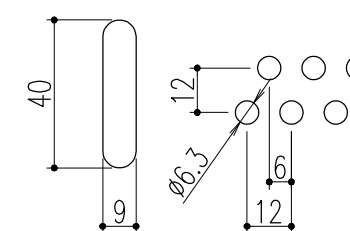
排水穴形状
