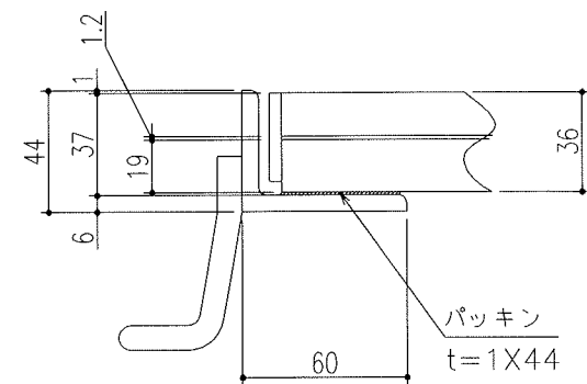
A部詳細図 S=1/3
