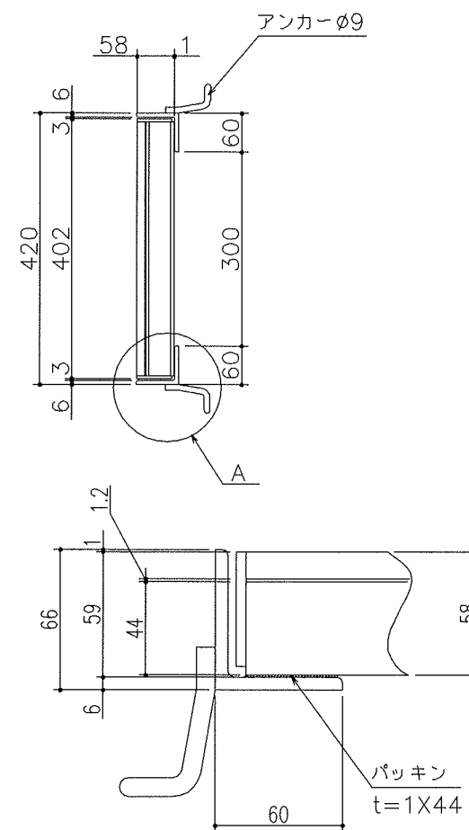
A部詳細図 S=1/3
