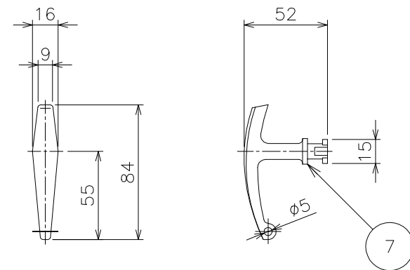
専用ハンドル詳細
