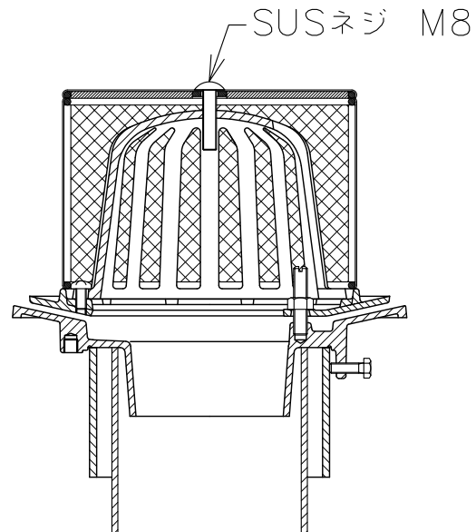
組図
