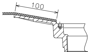
防水層の張り掛け幅は、100mm
