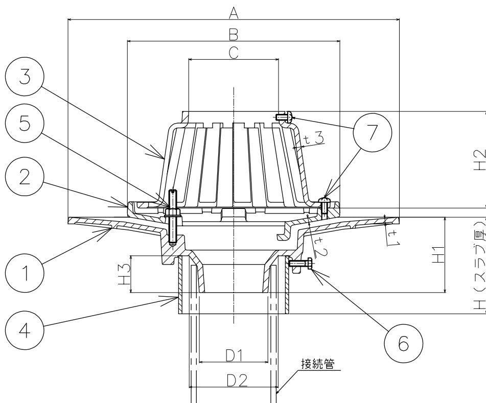
防水層張り掛け幅 100mm
