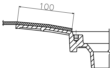
防水層張り掛け幅 100mm
