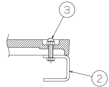
連結部断面
