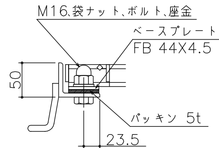
ボルト固定詳細図
