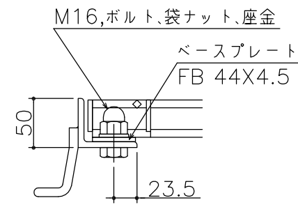
ボルト固定詳細図
