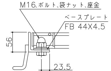
ボルト固定詳細図
