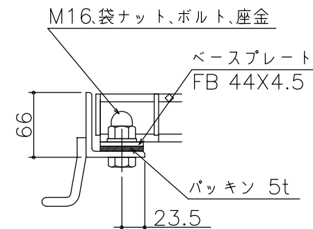
ボルト固定詳細図
