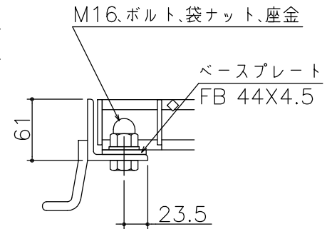
ボルト固定詳細図
