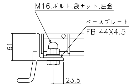
ボルト固定詳細図
