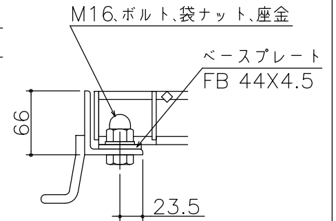
ボルト固定詳細図
