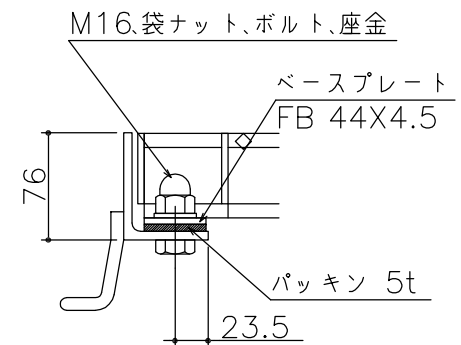
ボルト固定詳細図
