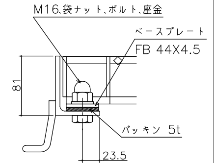
ボルト固定詳細図
