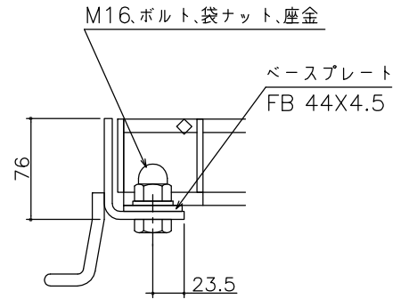
ボルト固定詳細図
