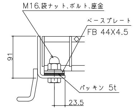
ボルト固定詳細図
