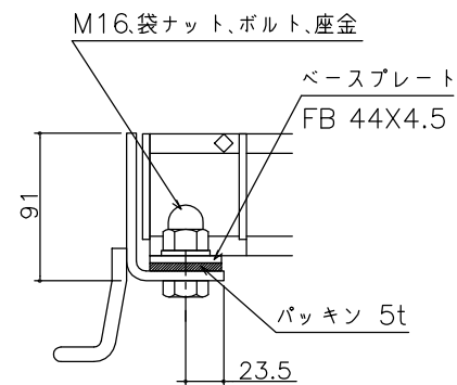
ボルト固定詳細図
