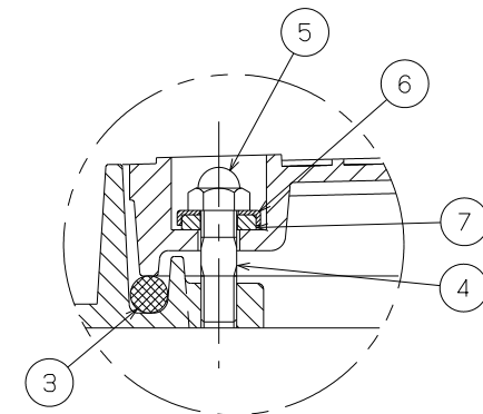
固定部拡大図
