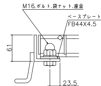
ボルト固定詳細図
