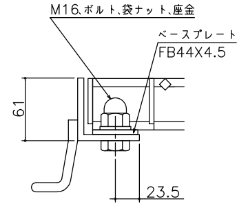
ボルト固定詳細図
