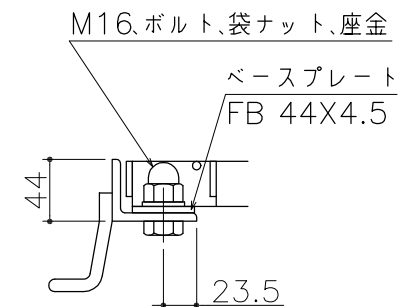
ボルト固定詳細図
