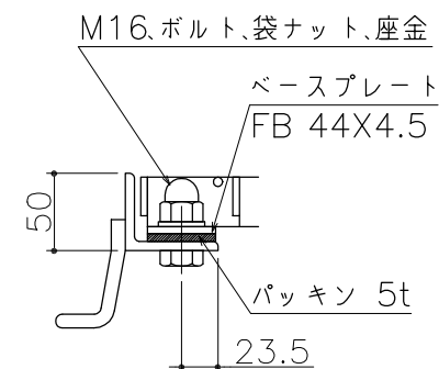
ボルト固定詳細図
