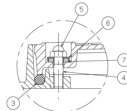
固定部拡大図
