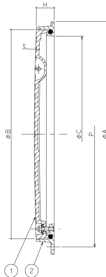
A-O-A断面図
