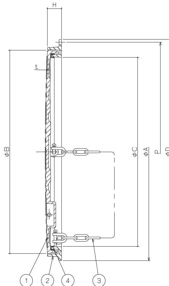
A-O-A断面図
