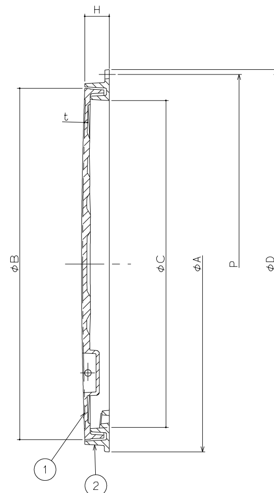
A-A断面図
