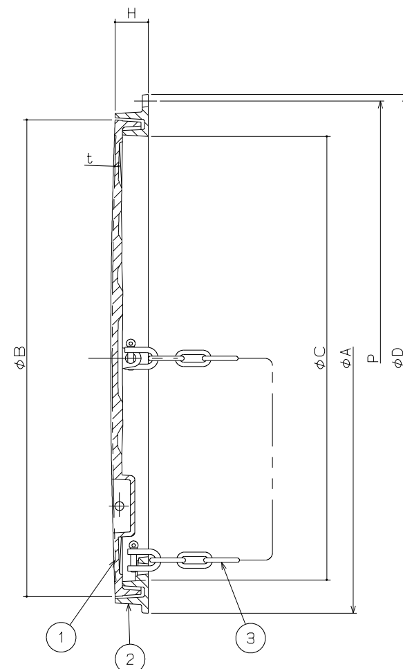
A-A断面図
