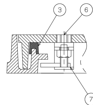
鉸部詳細図
