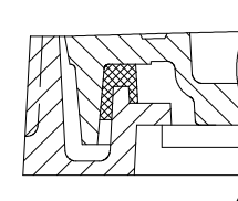
ロック部拡大図
