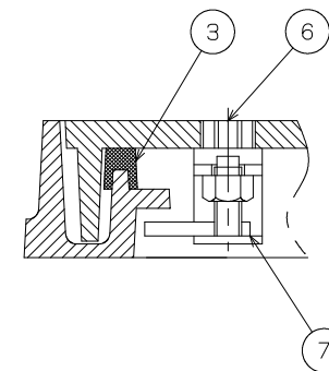
錠部詳細図
