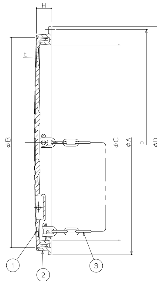
A-A断面図
