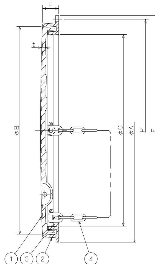
A-O-A断面図
