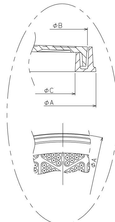
X部詳細 呼称300.350.400.500
