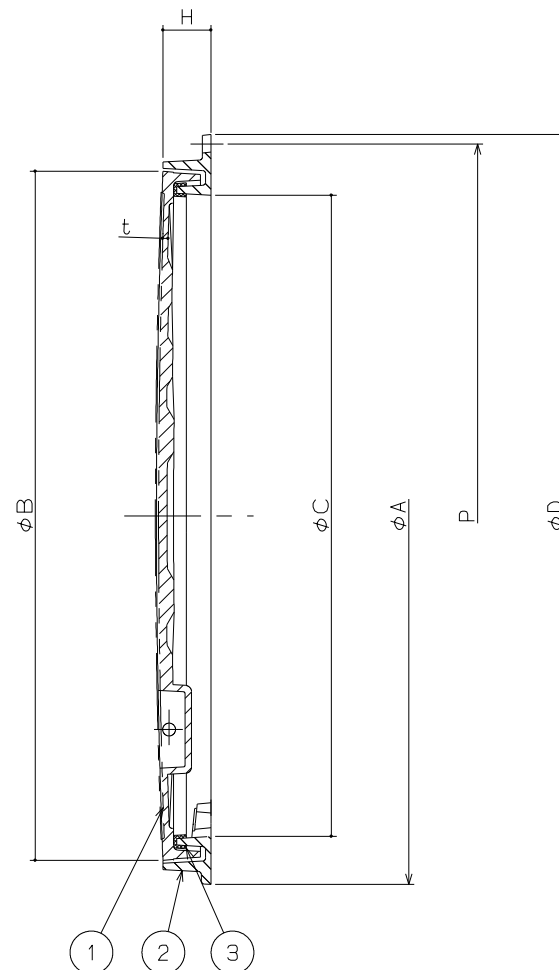
A-A断面図
