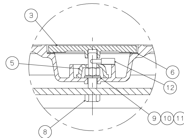
錠部拡大図
